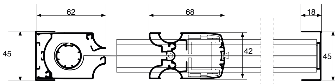
SEZ. ORIZZONTALE
