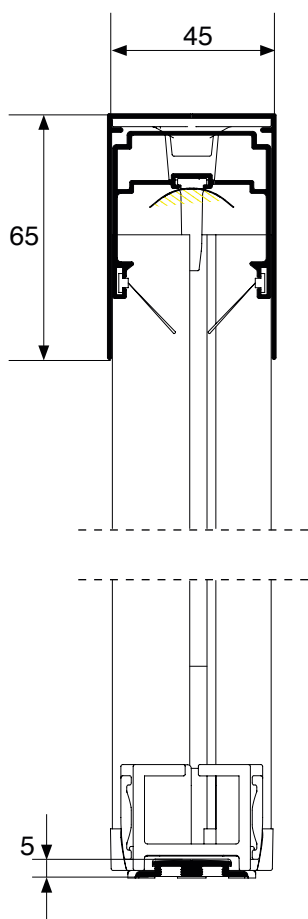
SEZ. VERTICALE
